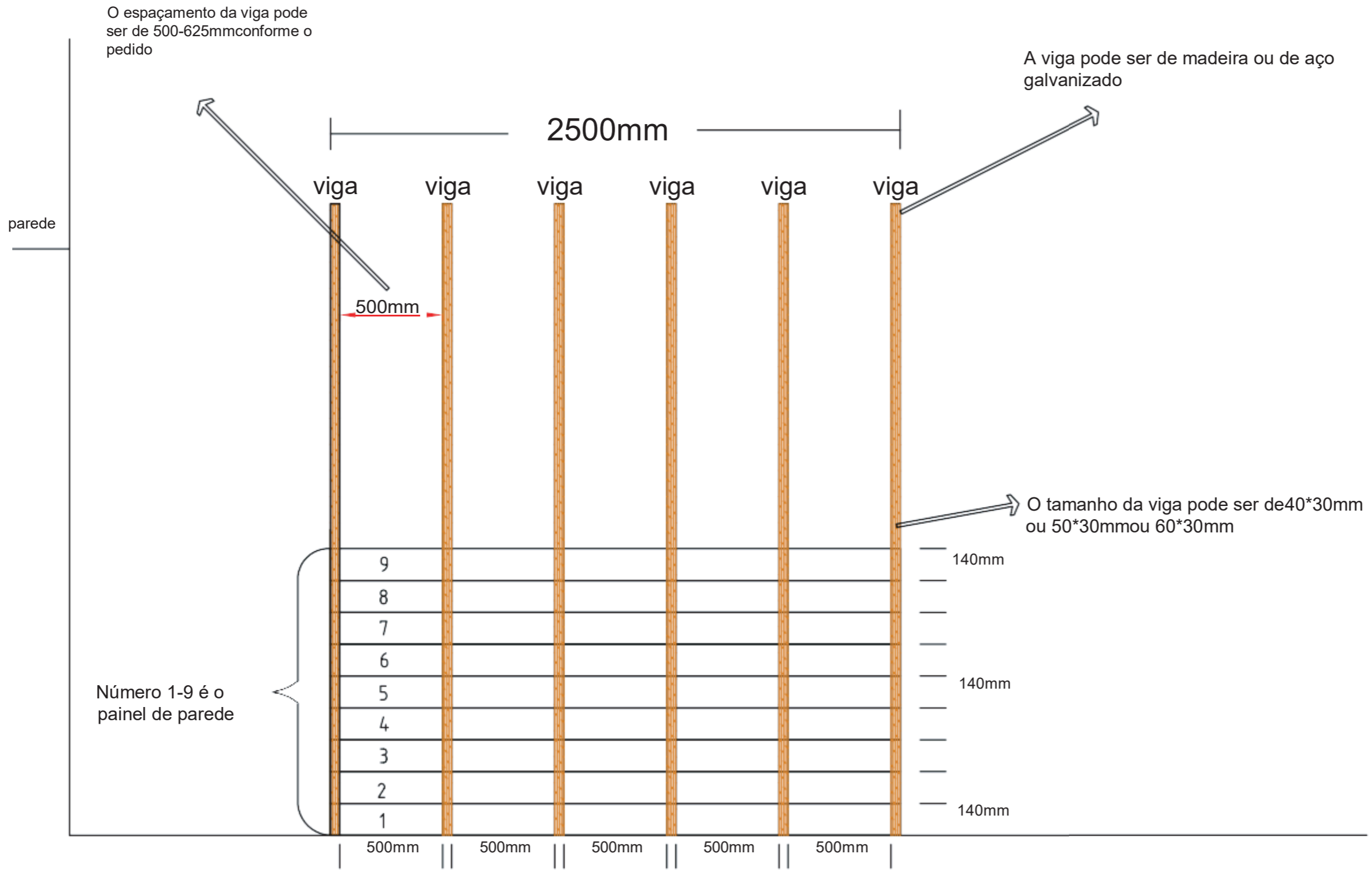
VISÃO FRONTAL DO PAINEL DE PAREDE (Desenho1)
