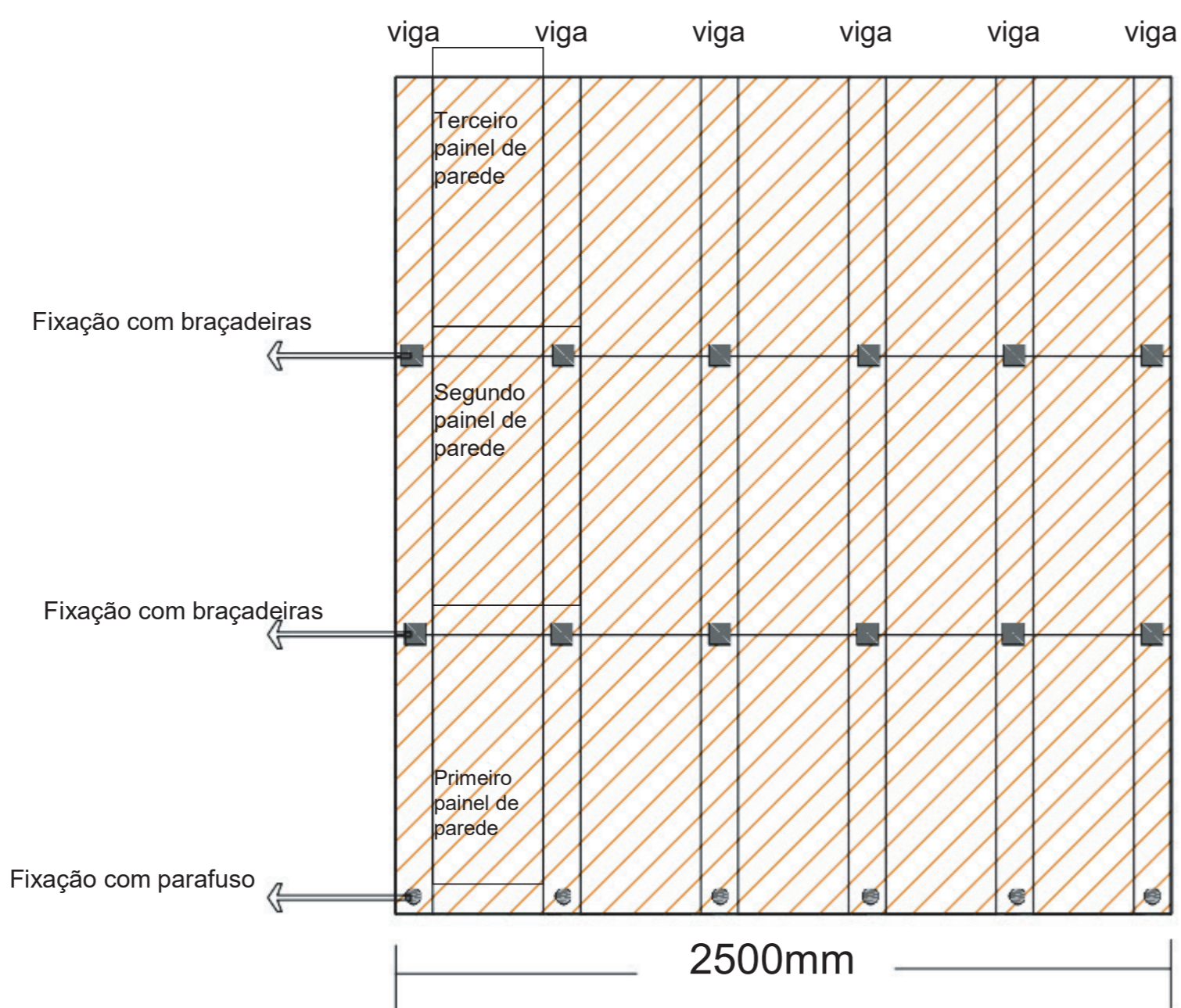
VISÃO FRONTAL AMPLIADA DO PAINEL DE PAREDE(Desenho2)
